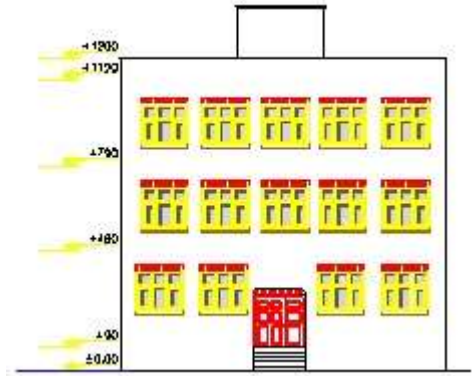
تصویر شماره ۱- طبقات و ارتفاع در ساختمان اداری
